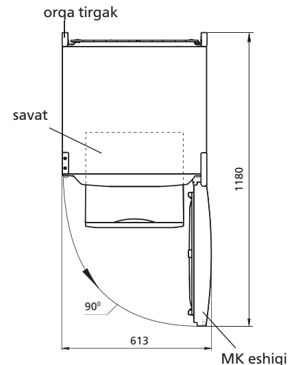
2 rasmi - Sovutgich (tepadan ko'rinish)
